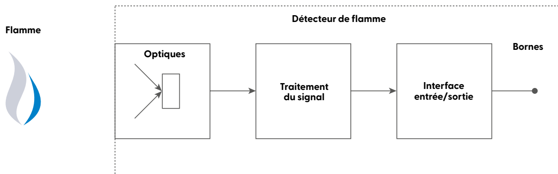
Figure 1. Schéma fonctionnel du traitement du signal du détecteur
