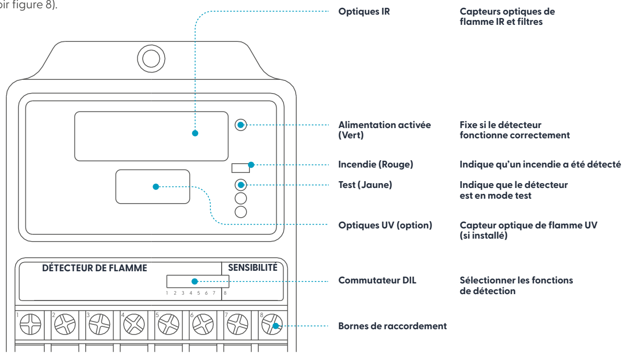
Figure 8. Détecteur avec couvercle avant retiré
