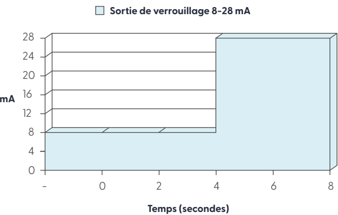
Figure 11. Réponse typique lorsqu'une flamme est détectée
