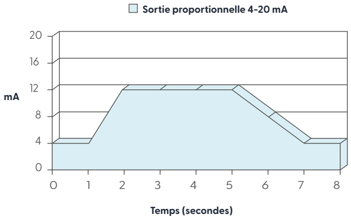
Figure 14. Réponse typique à une flamme soudaine
