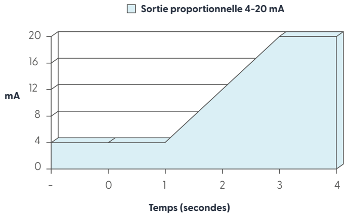
Figure 12. Réponse typique lorsqu'une flamme est détectée
