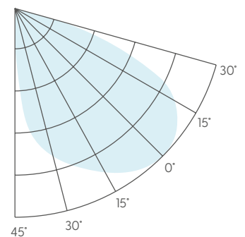
Figure 6. Portée relative en fonction de l'angle de vision horizontal (modèles à boîtier Ex d)
