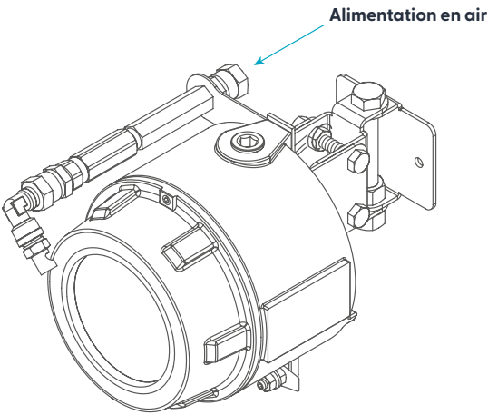
Figure 22. Kit d'épuration de l'air (12555)
