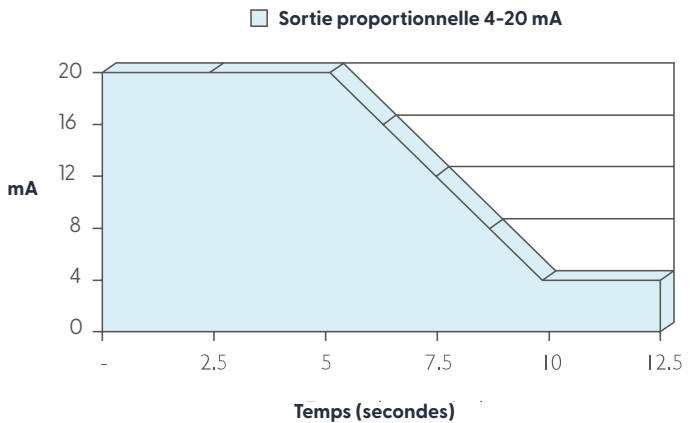
Figure 13. Réponse typique après la dernière flamme observée
