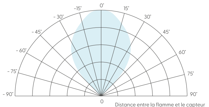
Figure 6. Portée relative en fonction de l'angle de vision horizontal (modèles à boîtier Ex d)
