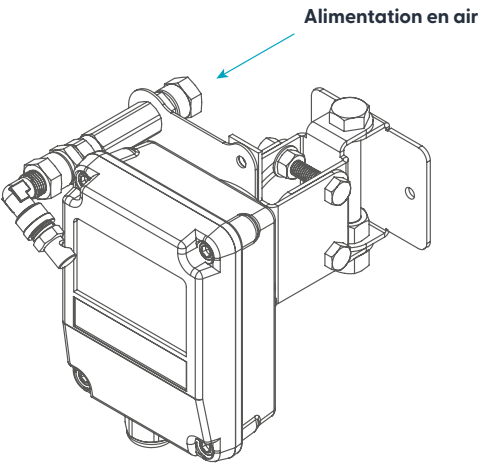
Figure 21. Kit d'épuration de l'air (12556)
