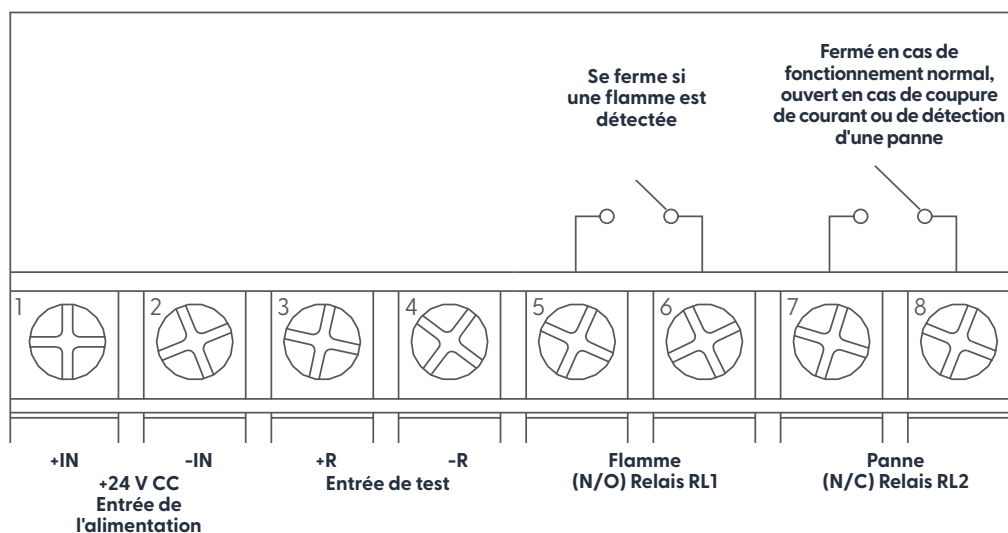
Figure 9. Bornes de raccordement électrique
