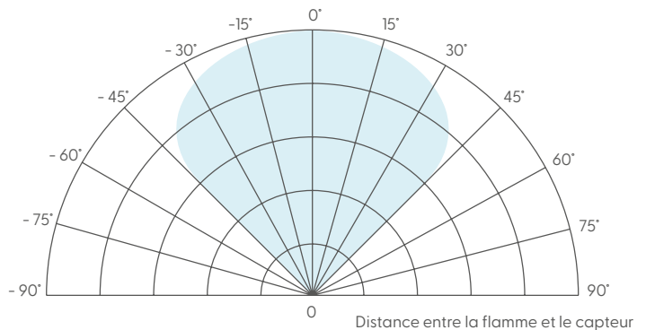
Figure 5. Portée relative en fonction de l'angle de vue (modèles à boîtier standard)
