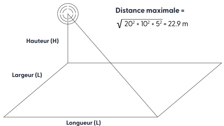
Figure 2. Calcul de la distance entre le détecteur et la flamme
