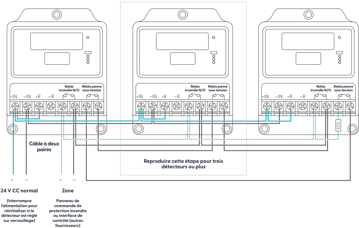
Figure 17. Schéma de connexion à quatre fils – détecteurs multiples
