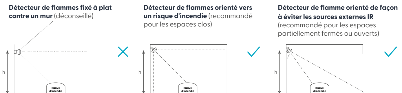
Figure 3. Placement du détecteur
